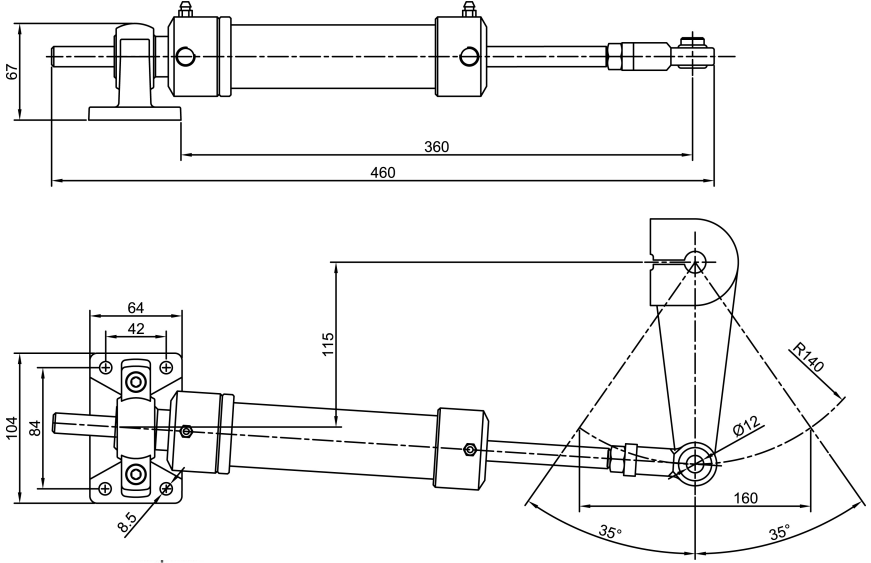
Şekil 1 (Drw.1)
