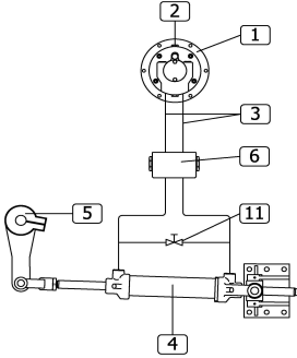
Şekil 3 (Drw.3)
