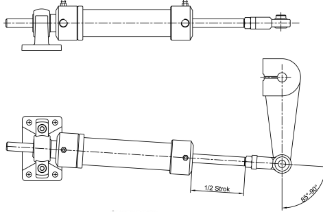
Şekil 2 (Drw 2)
