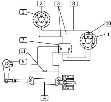
Şekil 4 (Drw.4)
