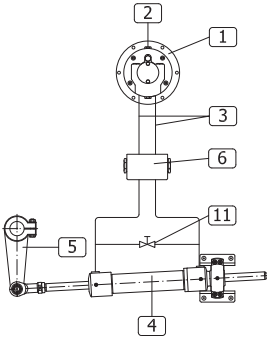
Şekil-3 (drw.3)
