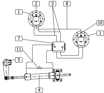
Şekil-4 (drw.4)
